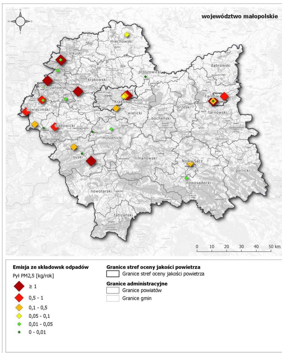
Rysunek 145. Emisja pyłu zawieszonego PM 2,5 ze składowisk odpadów w województwie małopolskim w 2018 r. 238
