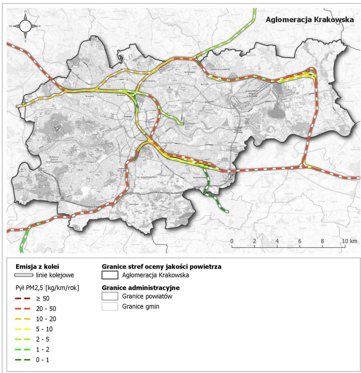
Rysunek 127. Emisja pyłu zawieszzonego PM 2,5 z innych źródeł (kolej) 220
