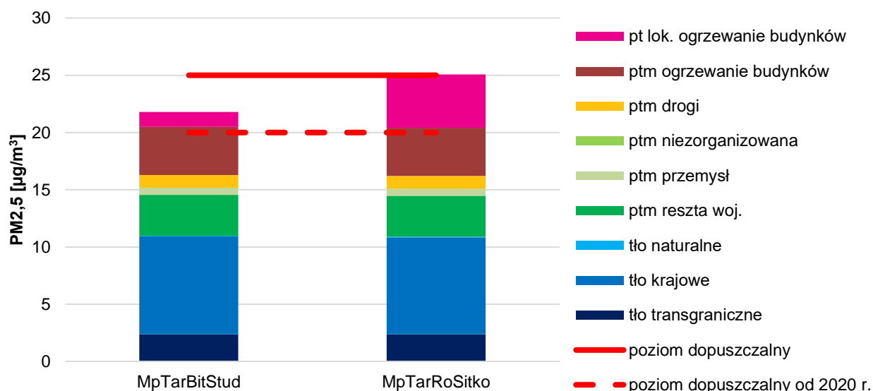
Rysunek 48. Prezentacja poziomów tła regionalnego, tła miejskiego oraz przyrostu tła lokalnego pyłu zawieszonych PM2,5 na stacjach pomiarowych w strefie miasta Tarnów w 2018 roku 88 .
