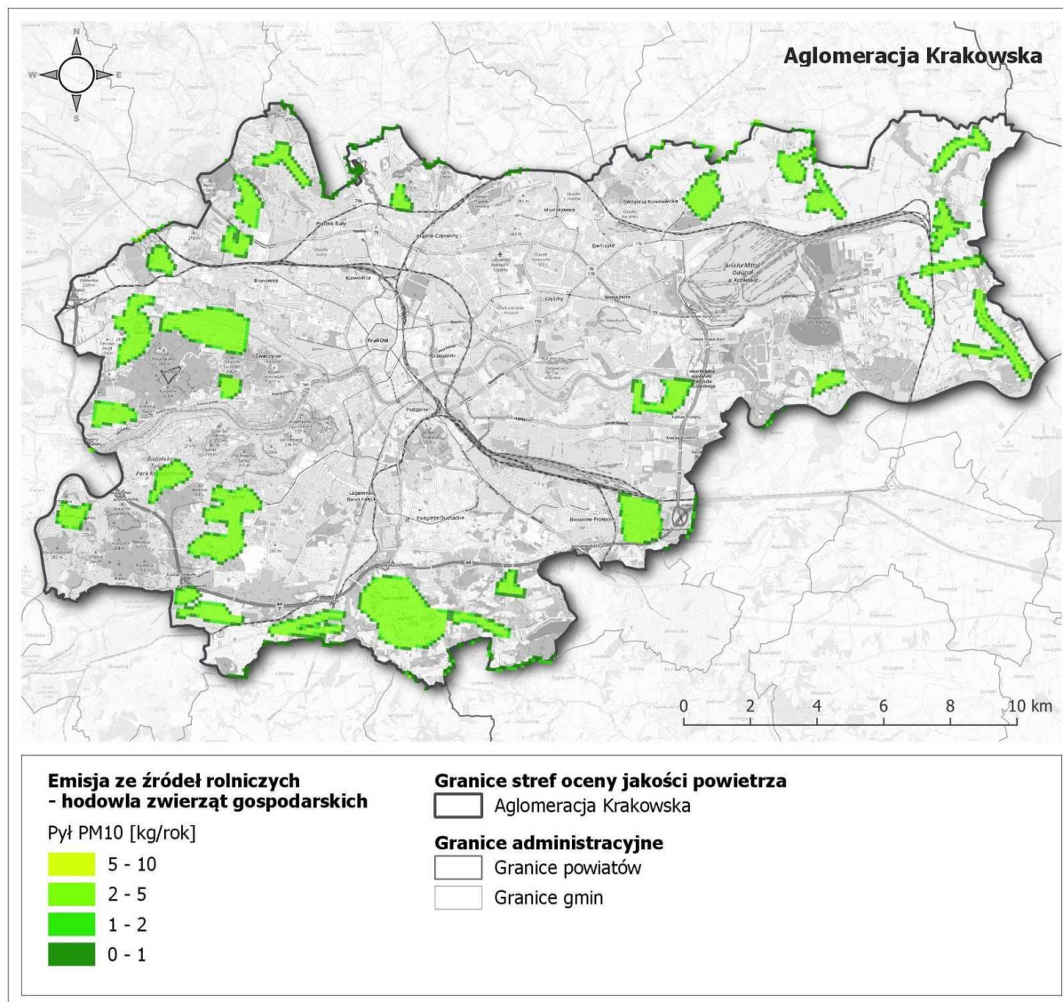
Rysunek 112. Emisja pyłu zawieszzonego PM10 ze źródeł rolniczych (hodowla) 205
