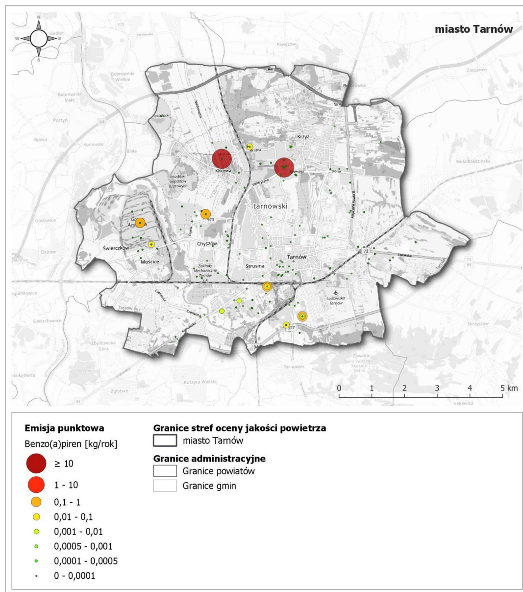
Rysunek 153. Emisja benzo(a)pirenu ze źródeł przemysłowych i energetycznych 246
