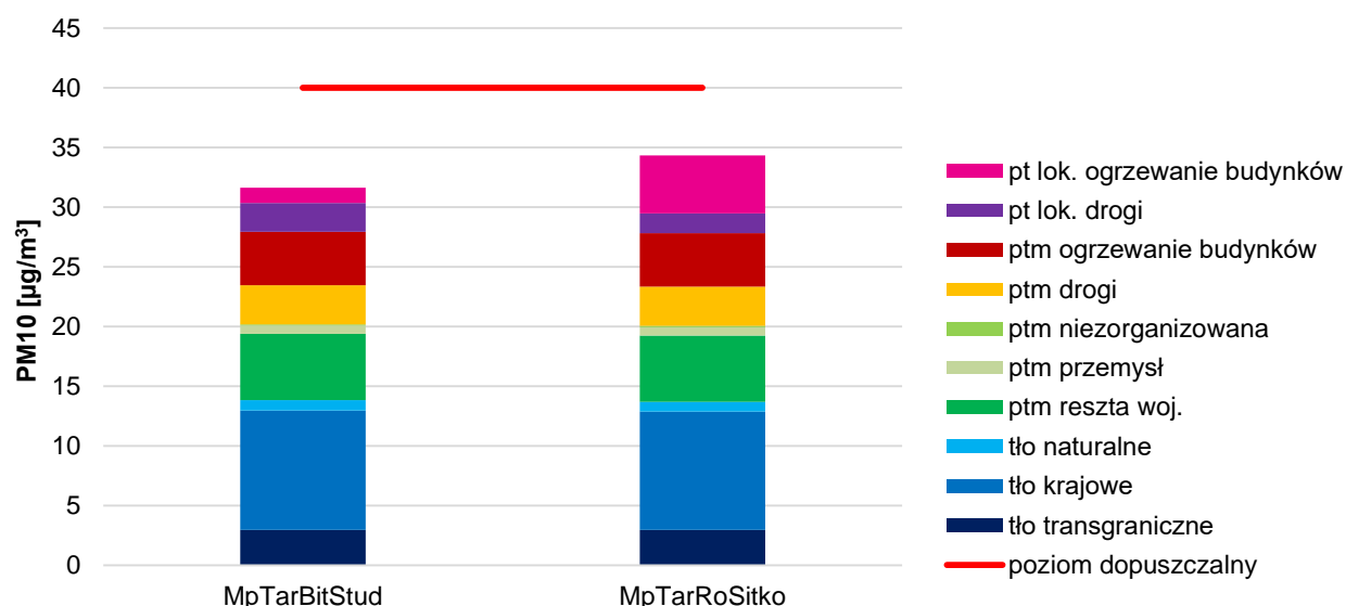
Rysunek 47. Prezentacja poziomów tła regionalnego, tła miejskiego oraz przyrostu tła lokalnego pyłu zawieszonego PM10 na stacjach pomiarowych w strefie miasta Tarnów w 2018 roku 86 .
