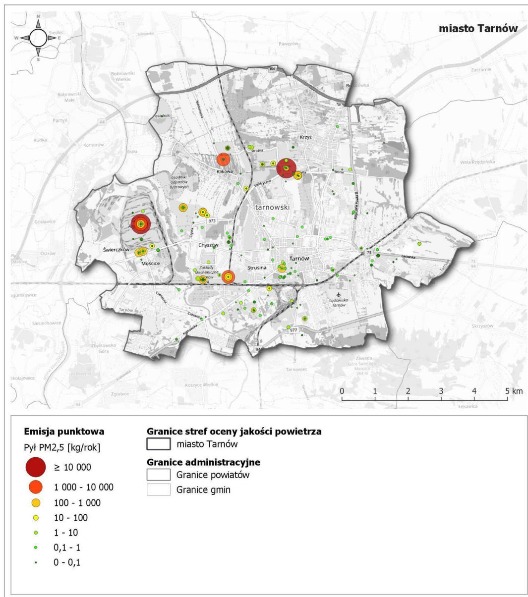
Rysunek 131. Emisja pyłu zawieszonego PM 2,5 ze źródeł przemysłowych i energetycznych 224
